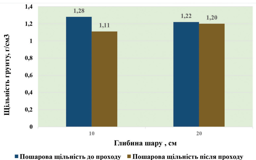
Рисунок 4 – Щільність ґрунту
