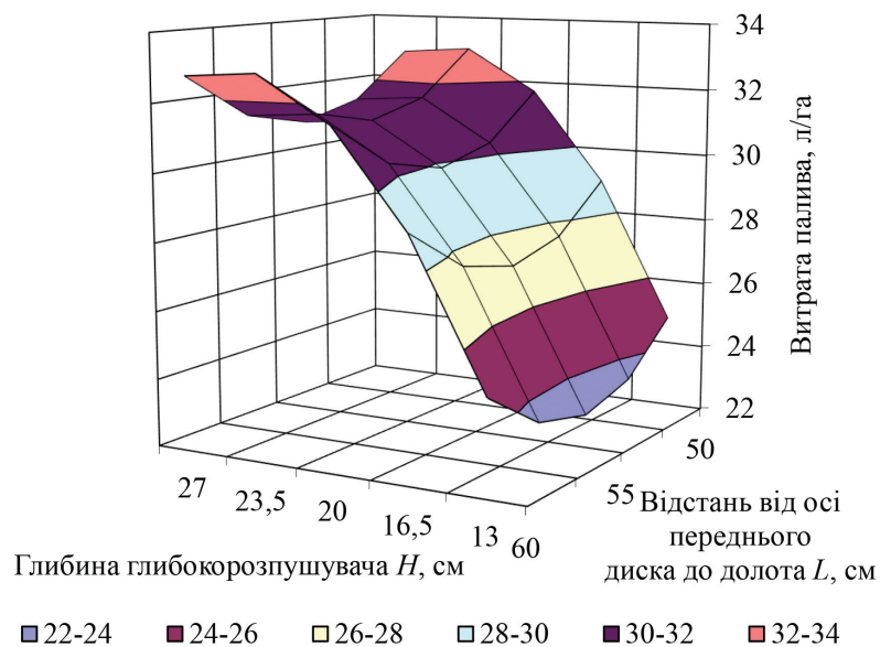
Рисунок 2 – Залежність витрати палива від глибини обробітку глибокорозпушувачем та від відстані від глибокорозпушувача до осі переднього диска за відстані від глибокорозпушувача до осі відрізних дисків C = 50 см
